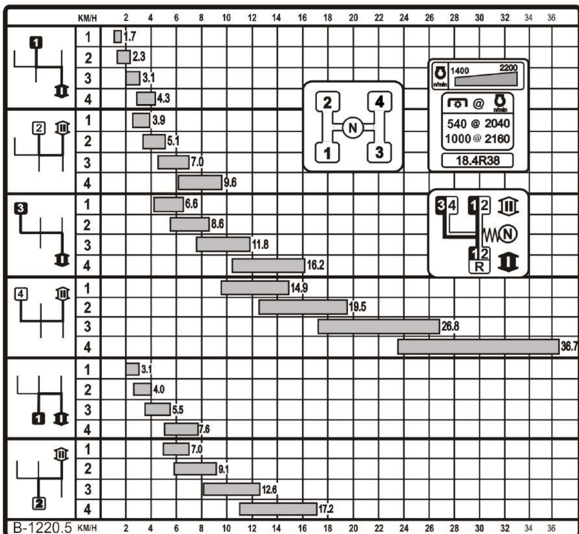
Рисунок 2.14.2 – Диаграмма скоростей трактора «БЕЛАРУС-1220.5» с КП 16x8
