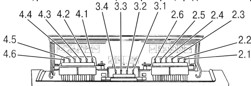
Рисунок 2.20.2 – Размещение предохранителей в щитке приборов
