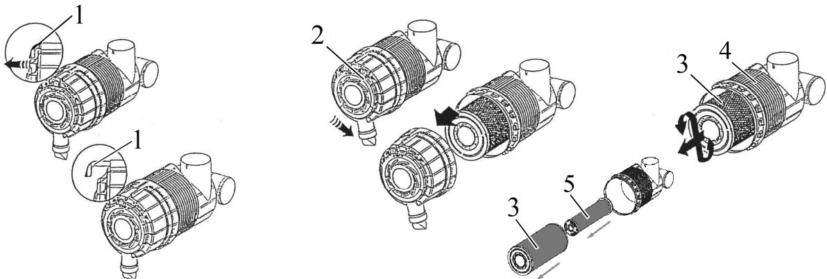
Рисунок 5.4.20 – Обслуживание воздухоочистителя дизеля
