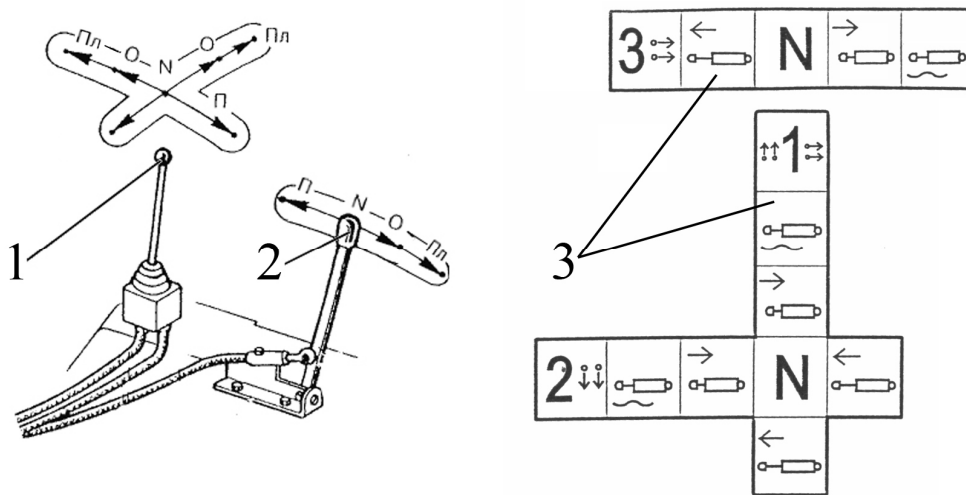
Рисунок 2.19.4 – Управление выносными гидроцилиндрами при установленном распределителе РП70-622 или РП70-622.1 посредством джойстика и рычага
