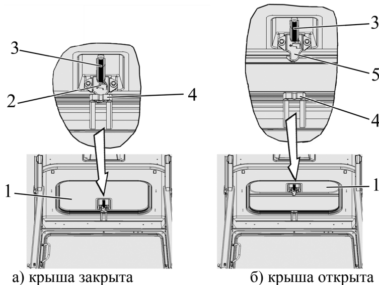
а) крыша закрыта б) крыша открыта 1 – крыша; 2 – зацеп; 3 – поручень; 4 – кронштейн; 5 – защелка.
