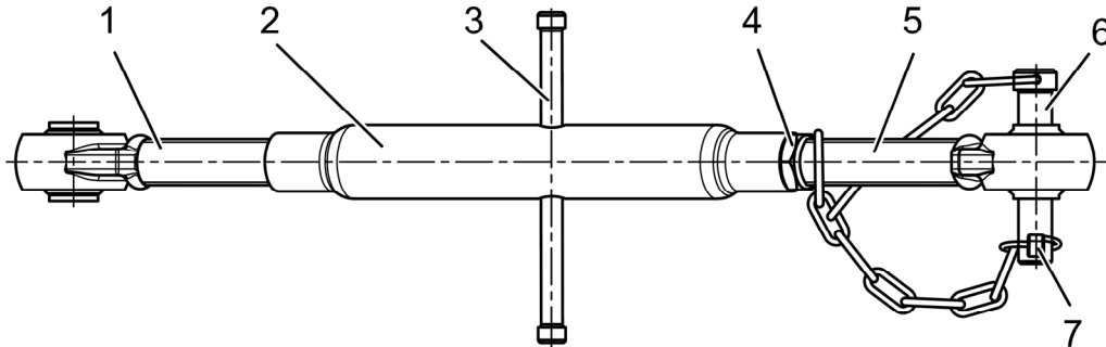
Рисунок 4.3.6 – Верхняя тяга
