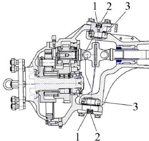
Рисунок 5.4.13 – Смазка подшипников осей шкворней ПВМ
