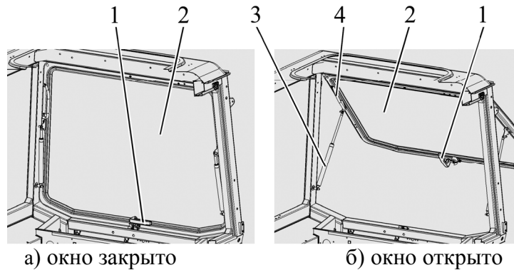
а) окно закрыто б) окно открыто 1 – рукоятка; 2 – заднее окно; 3 – пневмоподъемник; 4 – поручень.
