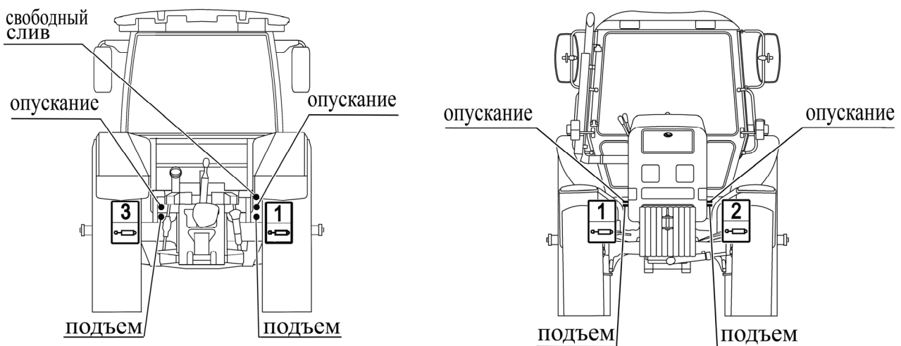
Рисунок 2.19.5 – Схема расположения и подключения выводов распределителя РП70-622 и РП70-622.1 к внешним потребителям
