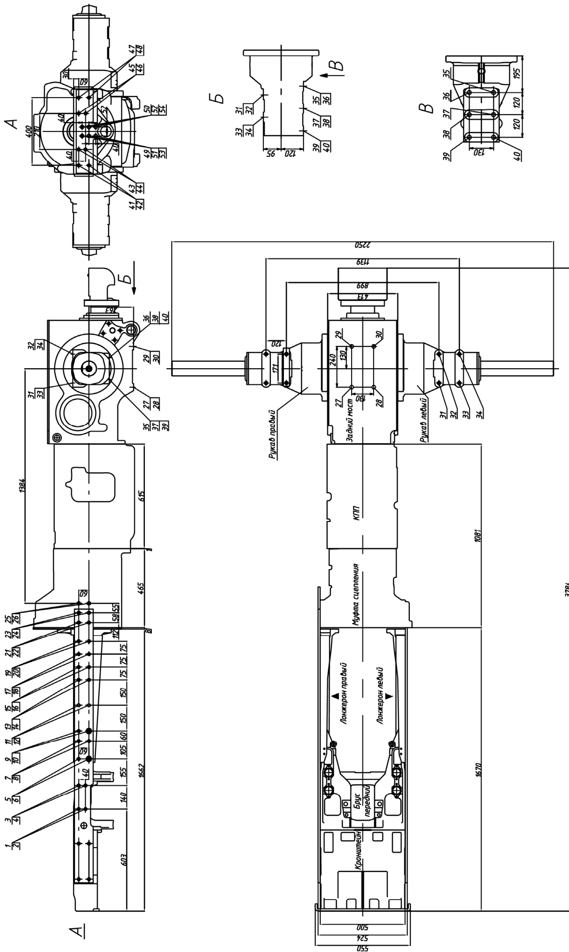
Рисунке 4.13.2 – Схема расположения монтажных отверстий трактора «БЕЛАРУС-1220.5»
