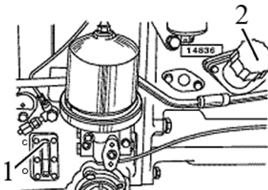
Рисунок 5.4.2 – Проверка уровня масла в трансмиссии
