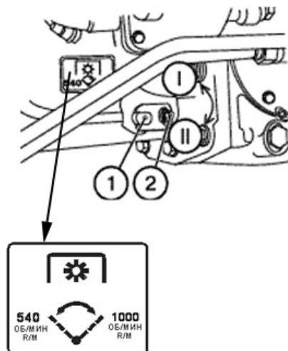
1 – поводок; 2 – болт.
