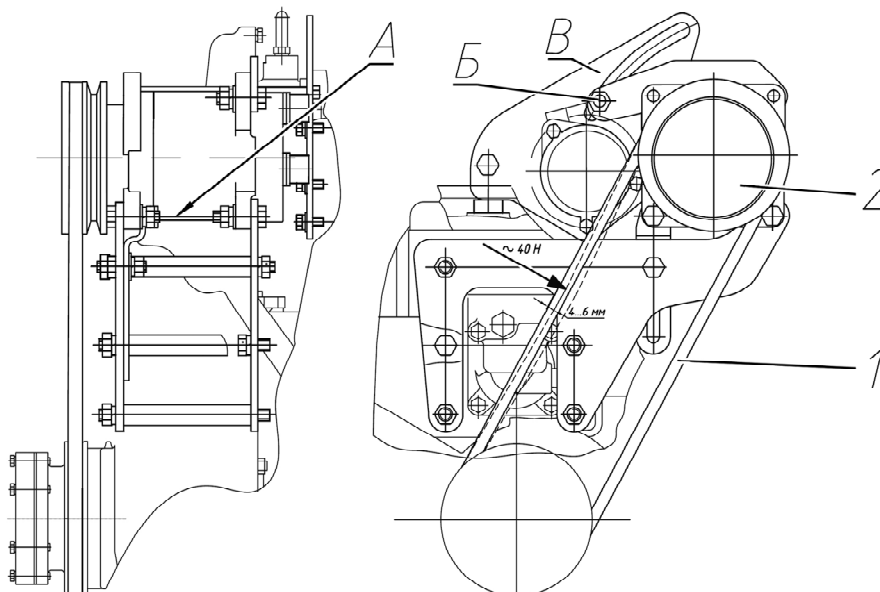
Рисунок 5.4.14 – Регулировка натяжения ремня привода компрессора кондиционера
