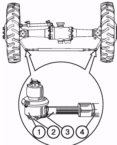
Рисунок 5.4.16 – Техническое обслуживание шарниров рулевых тяг
