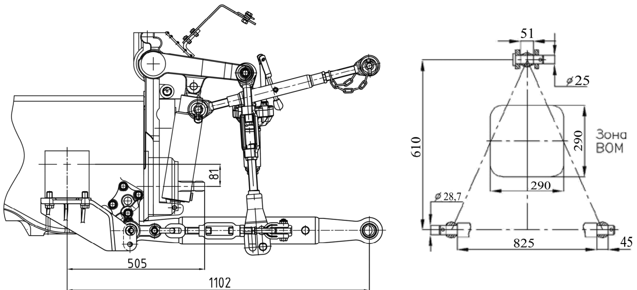
Рисунок 4.3.1 – Схема заднего навесного устройства исполнения НУ-2
