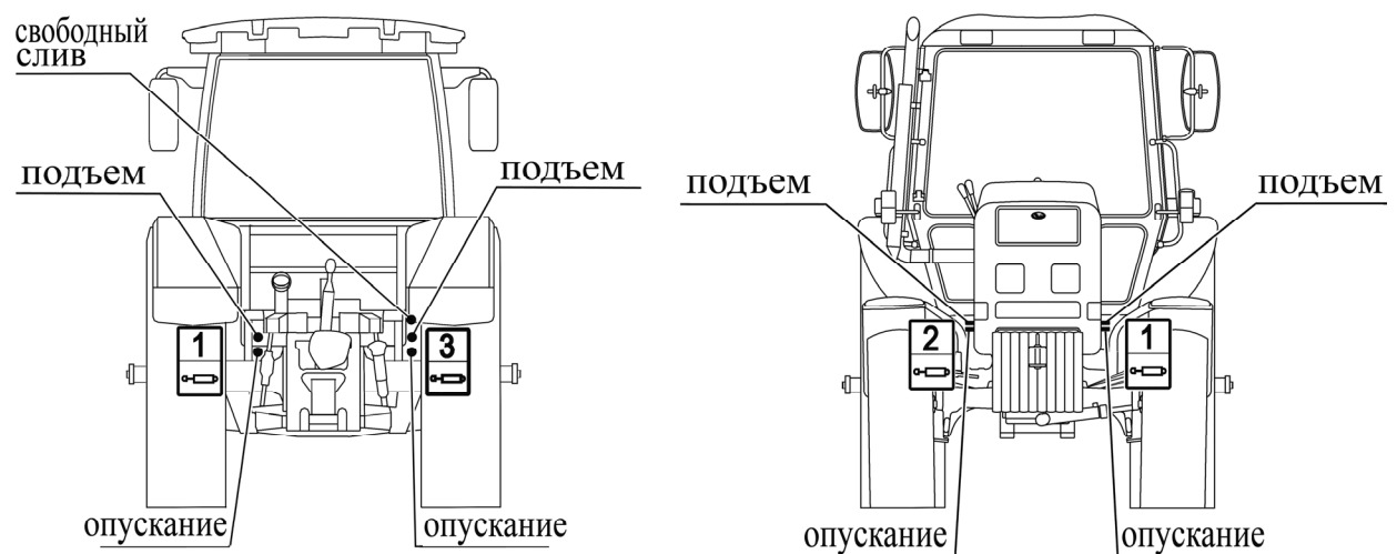
Рисунок 2.19.3 – Схема расположения и подключения выводов распределителя RS213Mita к внешним потребителям
