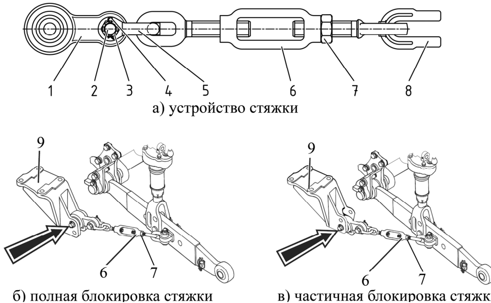
Рисунок 4.3.3 – Стяжка
