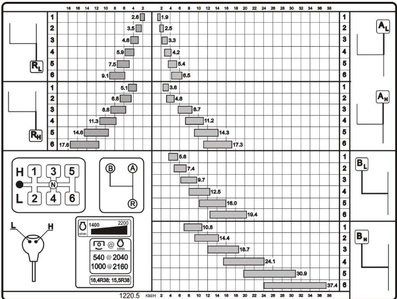
Рисунок 2.27.2 – Диаграмма скоростей трактора «БЕЛАРУС-1220.5» с КП 24х12
